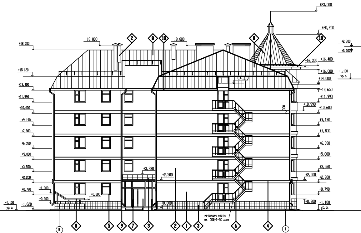
Фасад 8-1
