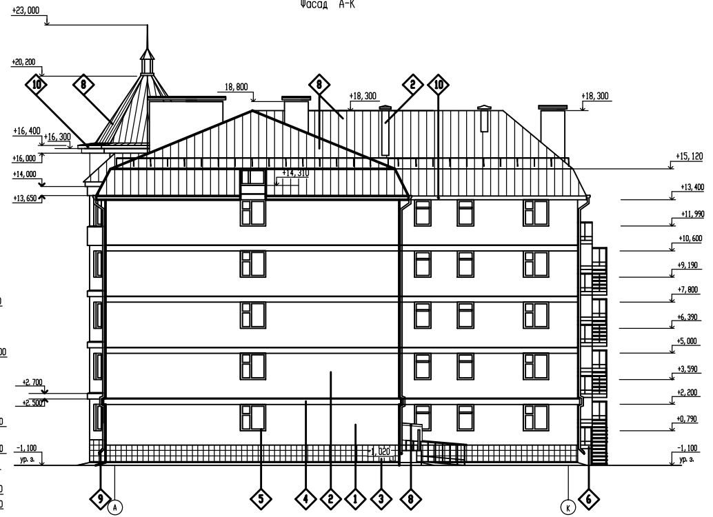
Фасад А-К
